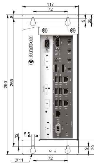
KBox C104-TGL-0
