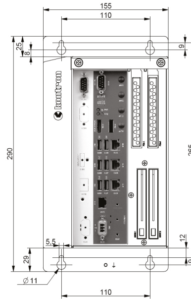
KBox C104-TGL-2
