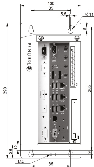
KBox C104-TGL-1
